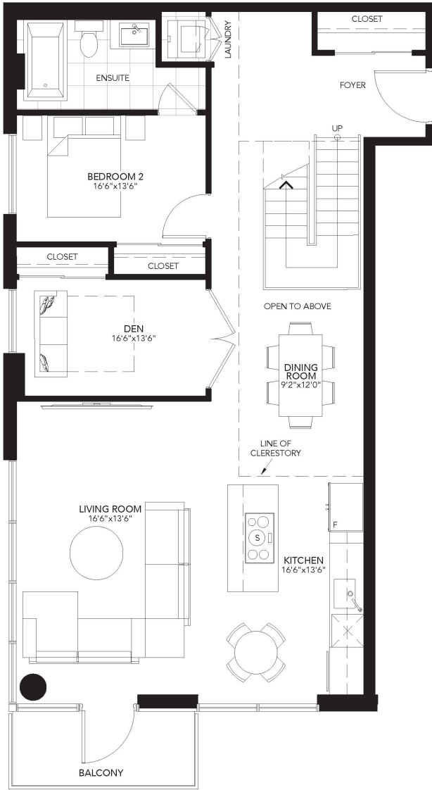
F10 LEVEL
