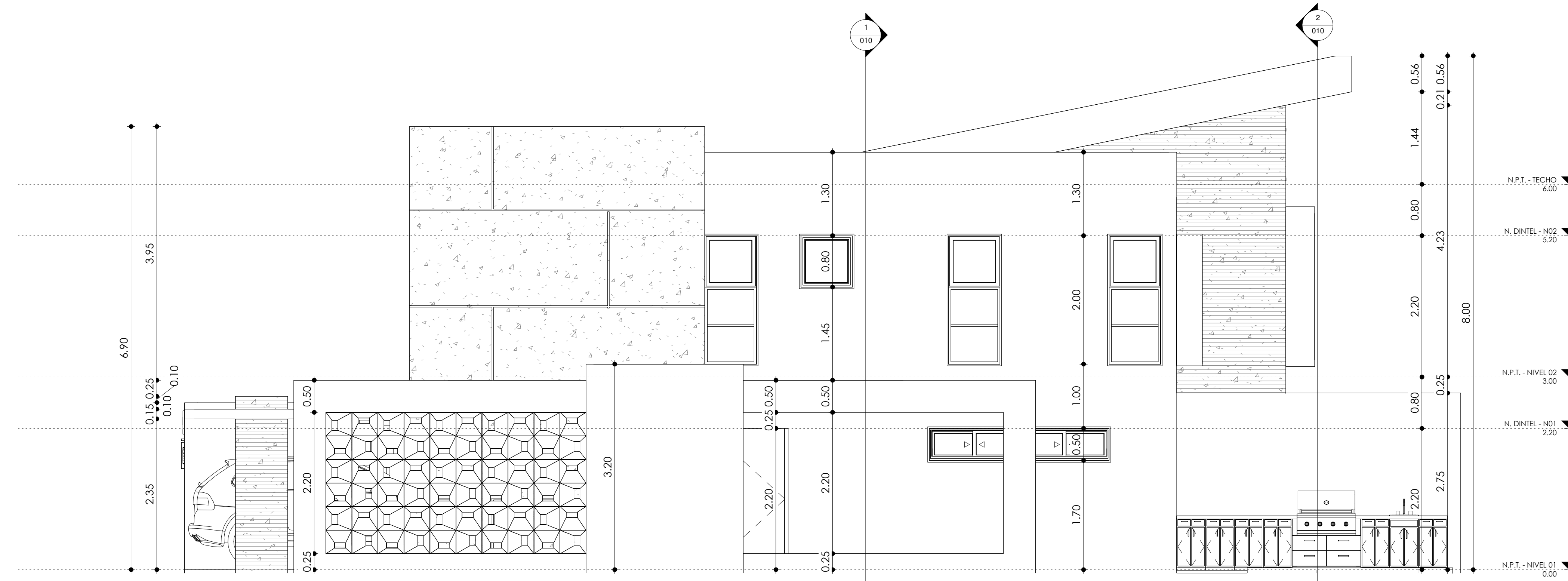
2 ELEVACION LAT. DERECHA 1:40
