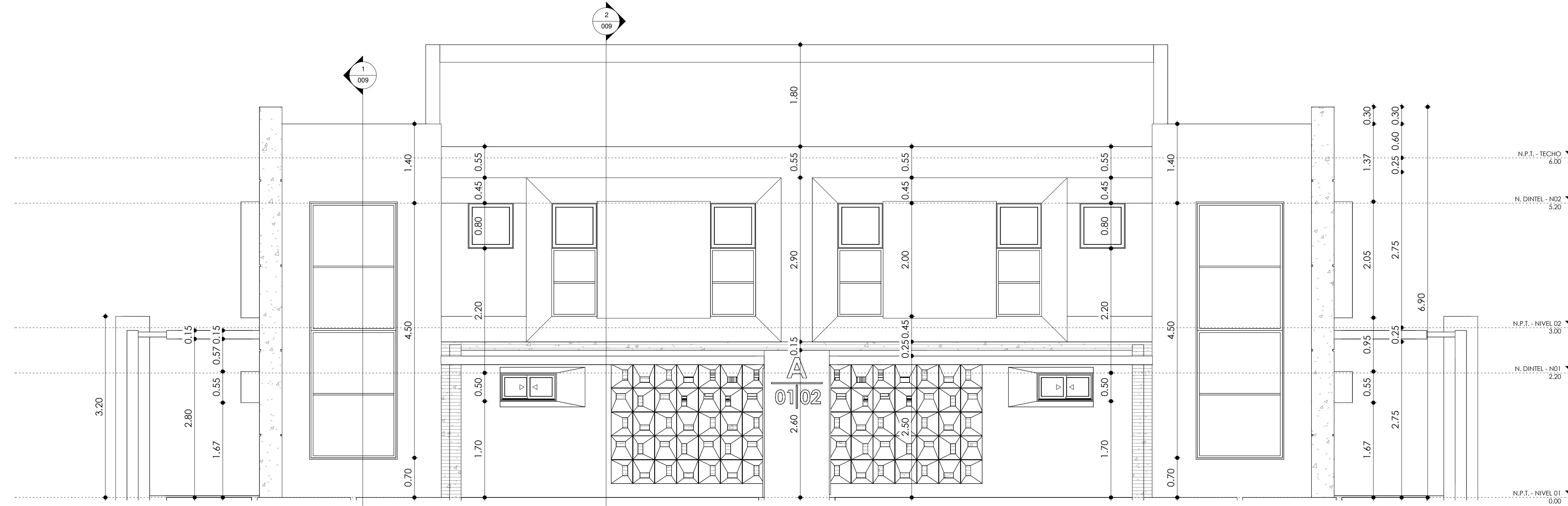
1 ELEVACION FRONTAL 1:40
